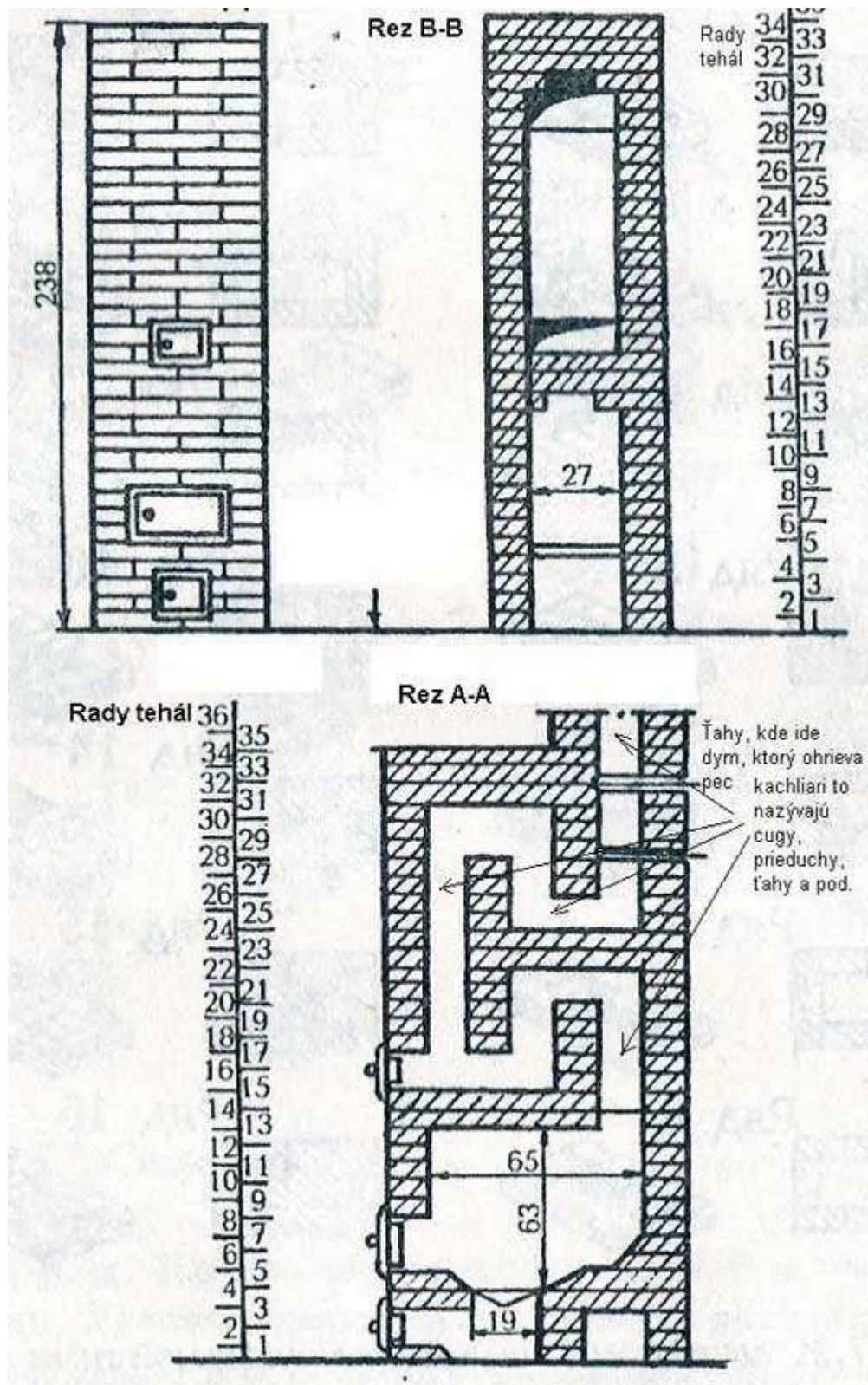
Pohľad na pec
